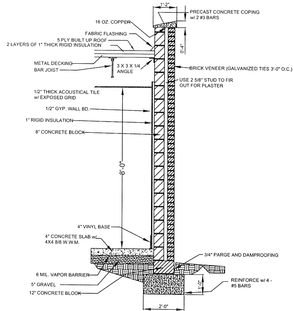
1 SECTION SCALE:
