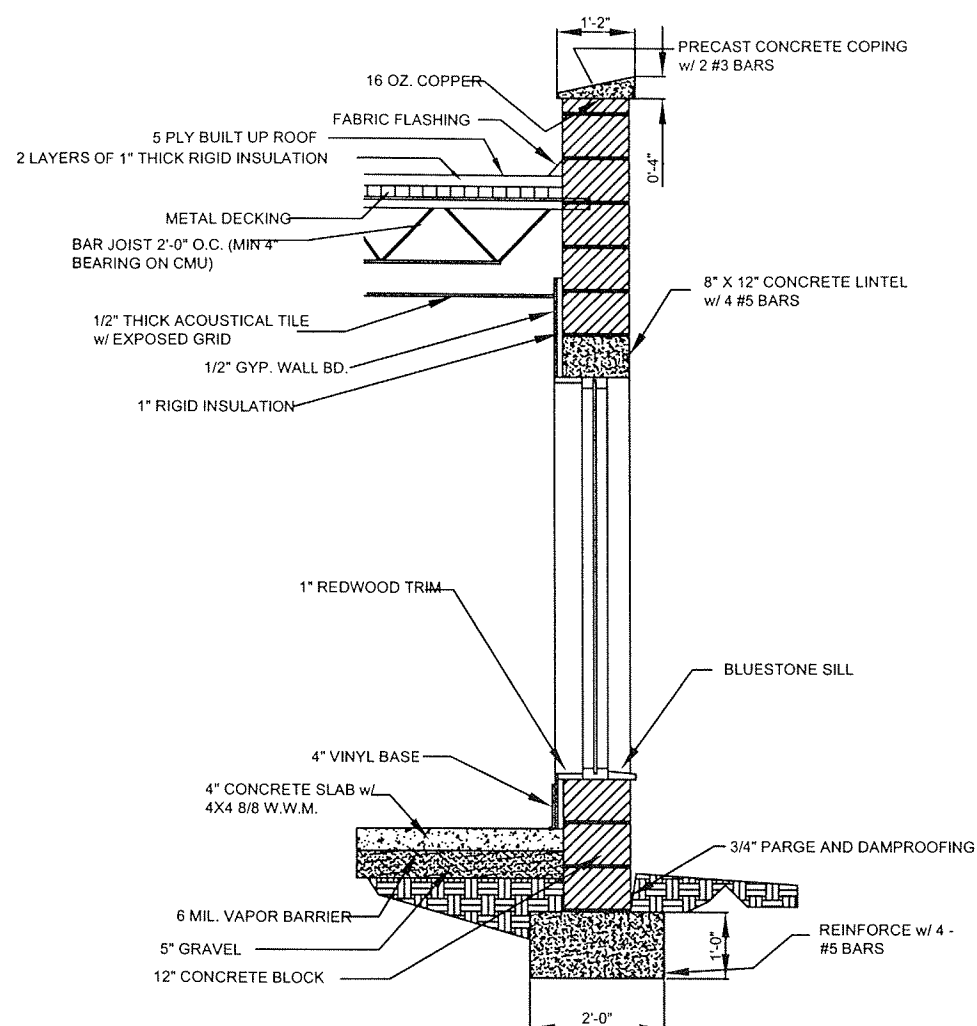
2 SECTION SCALE:
